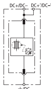
Prinzipschaltbild DSE M 1 60
