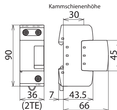
Maßbild DSE M 1 60
