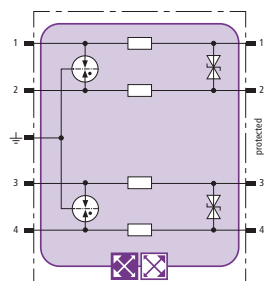
Prinzipschaltbild BXT ML4 BD 60
