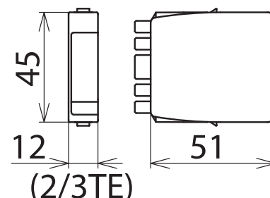
Maßbild BXT ML4 BD 60
