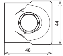
Maßbild
