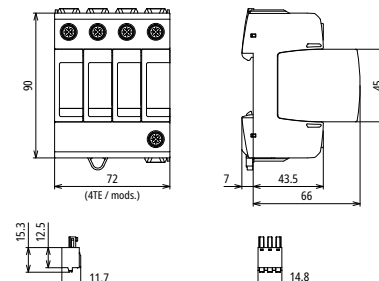
Maßbild DG MD TNS 150 FM
