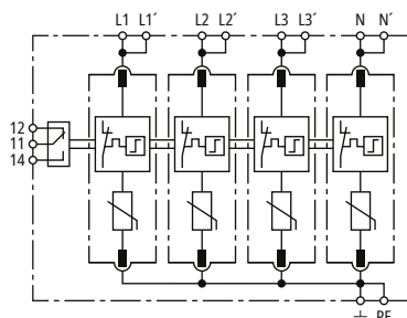
Prinzipschaltbild DG MD TNS 150 FM
