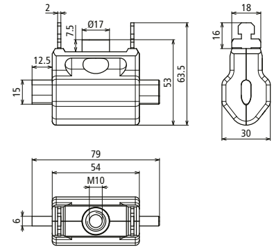
Maßbild EP NH00 TI SN7379
