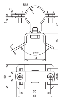
Maßbild LH ZS 27 30 SBH 25X0.3 V2A
