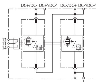
Prinzipschaltbild DSE M 2P 60 FM
