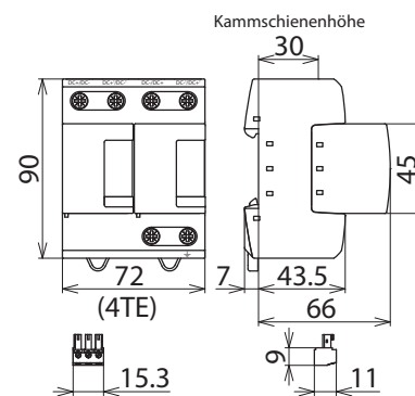
Maßbild DSE M 2P 60 FM
