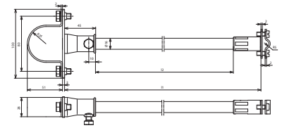
Maßbild DIDH 7.10 1030 D50 V2A
