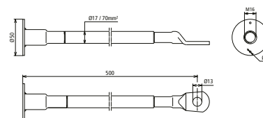
Maßbild D BEB 11 / EBS 15-03-27
