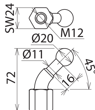
Maßbild KFP 20 W45 M12
