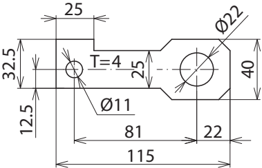
Maßbild AB EXFS IF3 G 22
