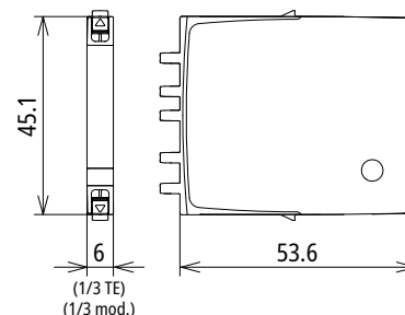
Maßbild BCO MOD ML2 BE HF 5
