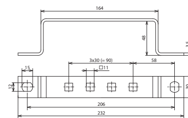
Maßbild ES 4AP 11X11 V2A
