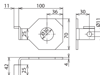
Maßbild AB EXFS IF1 W 30
