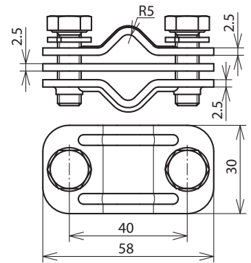
Maßbild UTK 200 2X10 FL30 ZP V2A
